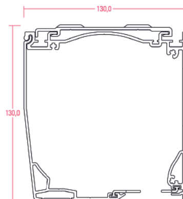
Cassetto di 130
