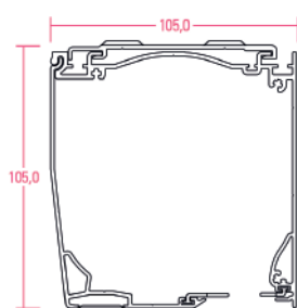
Cassetto di 105
