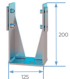
Verstellbare Stütze
