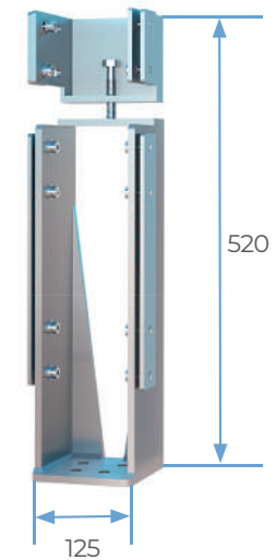
Verstärkte verstellbare Stütze
